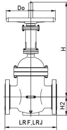
Исполнение RN19013 - шибер без проходного отверстия
