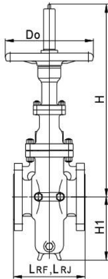
Исполнение RN19001 - шибер с проходным отверстием
