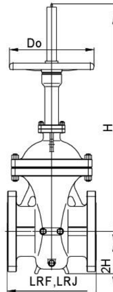
Исполнение RN19012 - шибер без проходного отверстия
