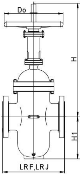
Исполнение RN19003 - шибер с проходным отверстием
