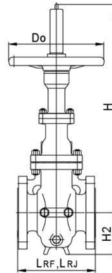
Исполнение RN19011 - шибер без проходного отверстия
