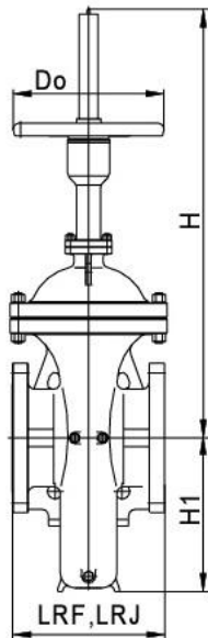
Исполнение RN19002 - шибер с проходным отверстием
